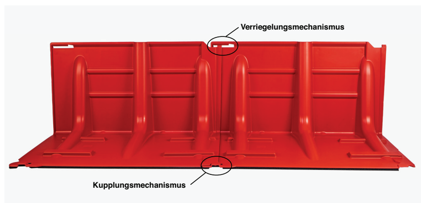
BW52 Kupplungs- und Verriegelungsmechanismus
