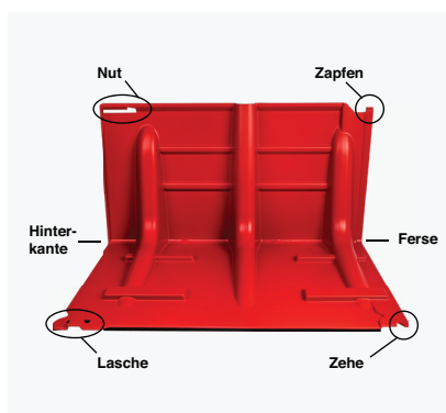
BW52 Teilebeschreibungen
